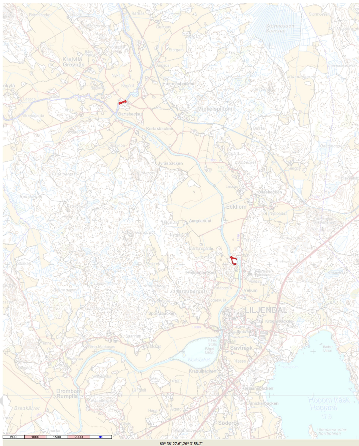
Kuva 3 Kaksi koskialuetta, Myrskylä ja Loviisa
