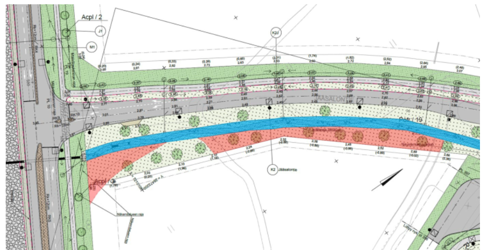
Kuva 2. Ote asemapiirroksista: punaisella viitasammakolle säästettävä kosteikkoalue ja sinisellä uusi Anttilanojan uoma.
