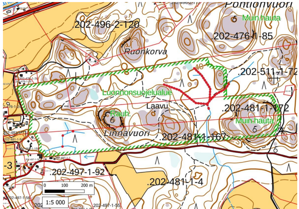
Kuva 1. Linnavuoren tukittavat ojat on merkitty punaisilla katkoviivoilla ja länsiosan kolme patoa on merkitty punaisilla pisteillä
