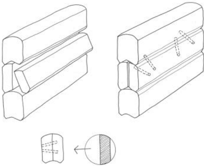
Kuva 21: Laho hirsi korjataan lankkupaikkauksella.
