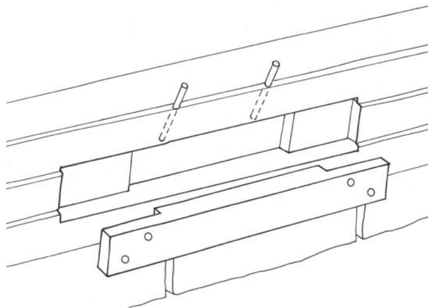
Kuva 27: "Pölkkyvarausta" voidaan käyttää hirren paikkaukseen silloin, kun rakennusta ei voida nostaa.
