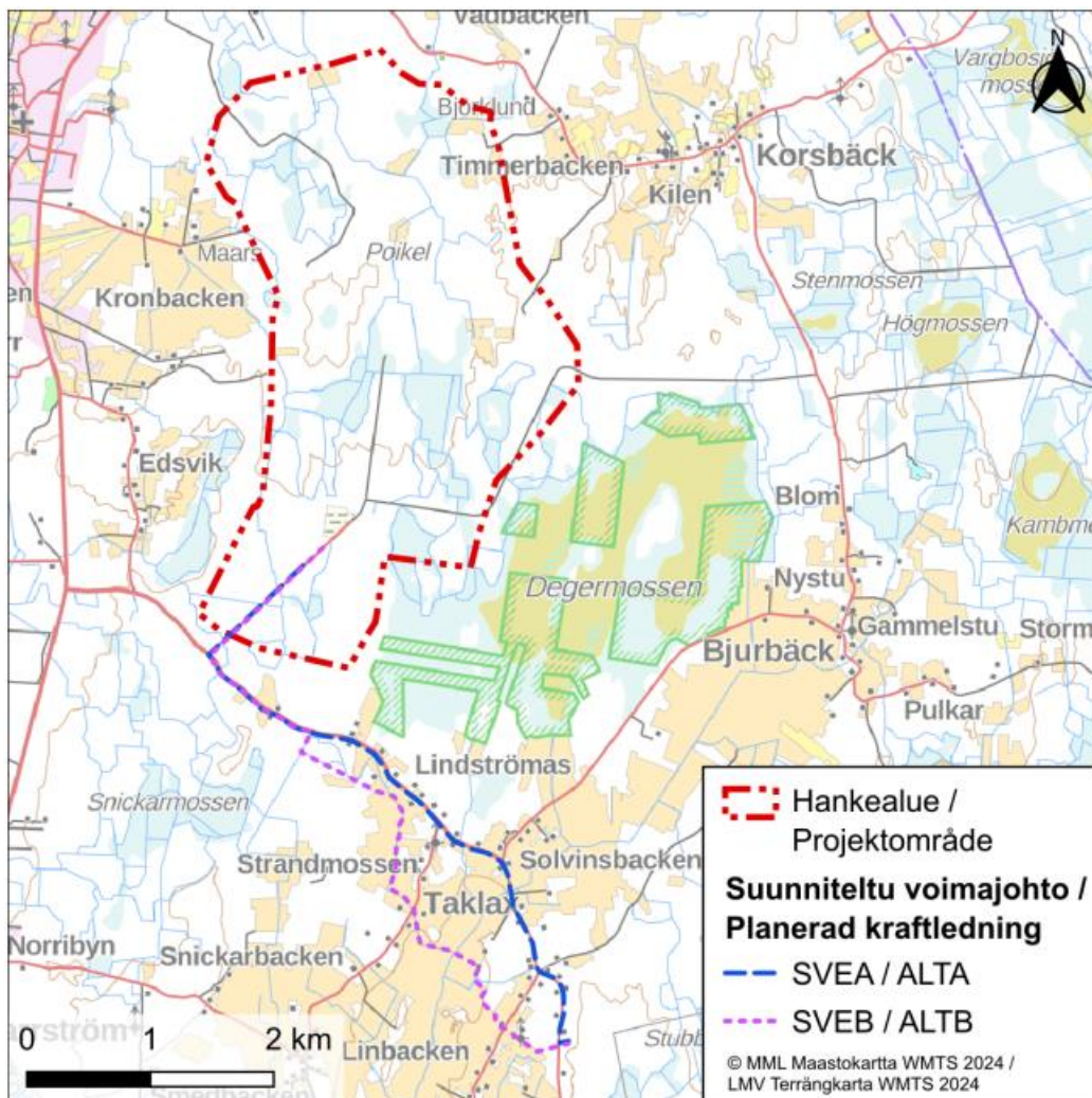
Kuva: Hankealue ja tarkasteltavat sähkönsiirtovaihtoehdot (kuva: FCG Rakennettu Ympäristö Oy).
