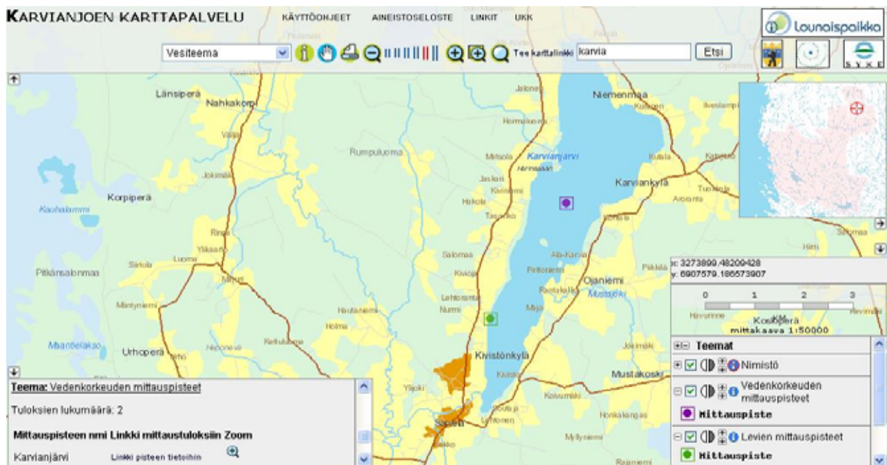
Kuva 2: Kuvakaappaus karttapalvelusta
