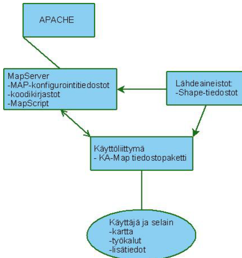
Kuva 1: Palveluarkkitehtuuri
