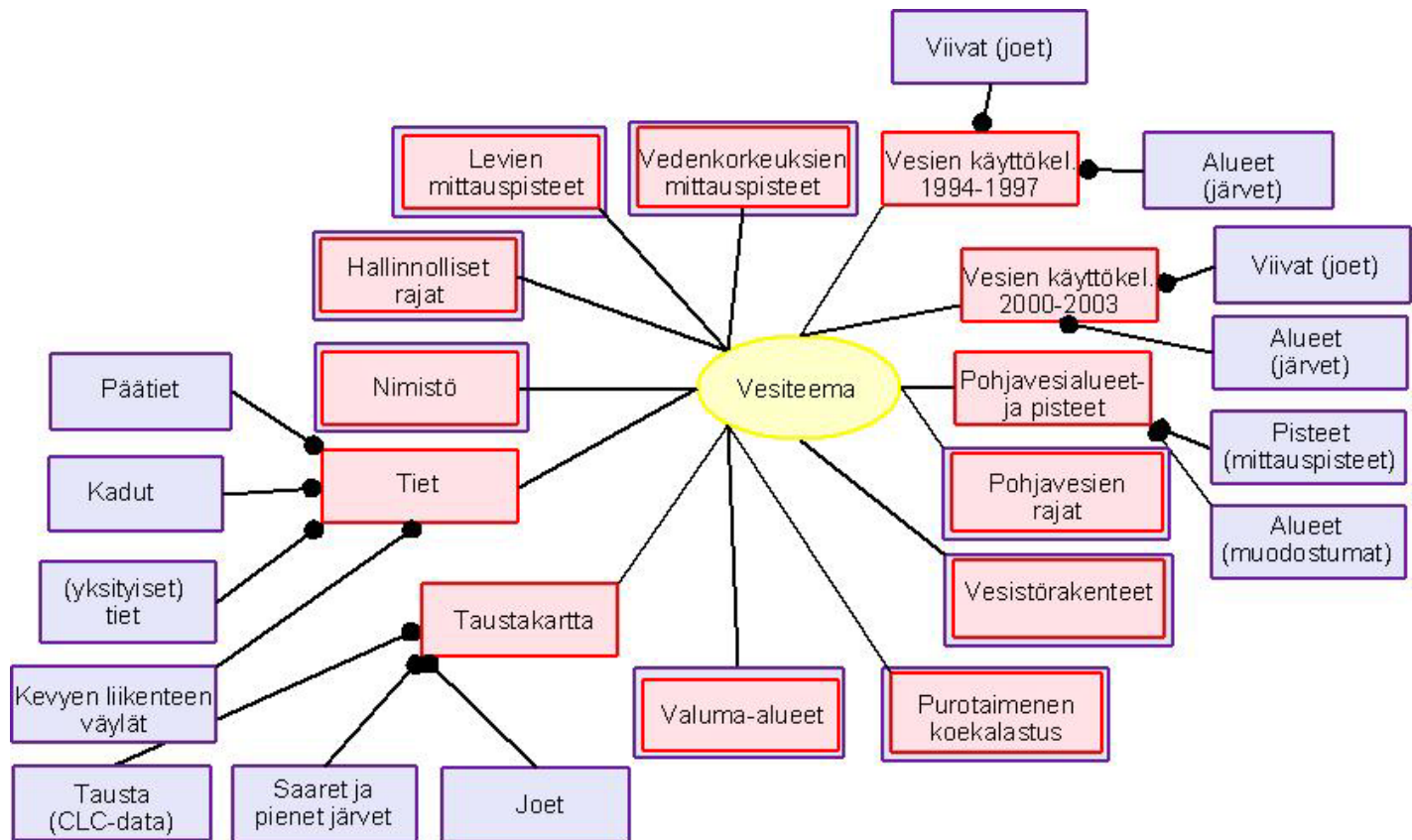
Kuva 3: Vesiteeman sisältö
