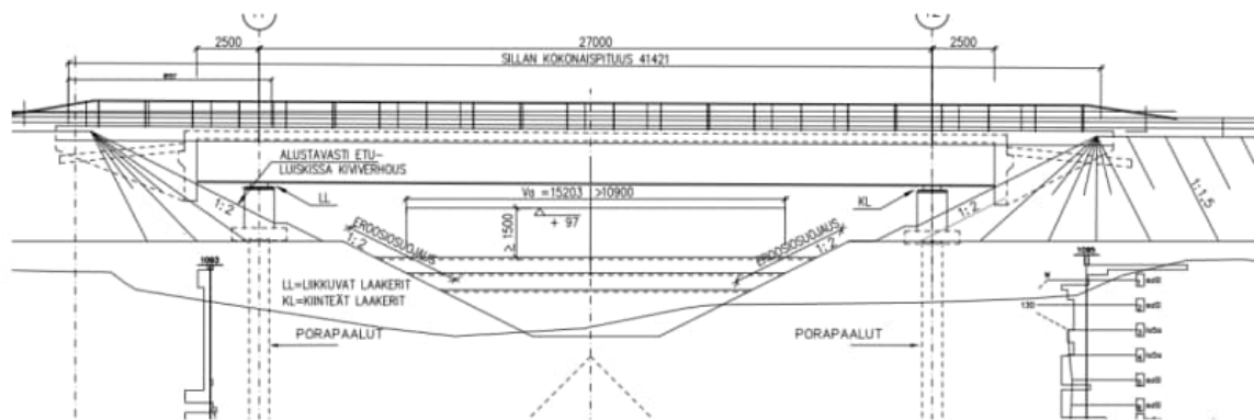
Kuva: 4 Liittopalkkisilta.
