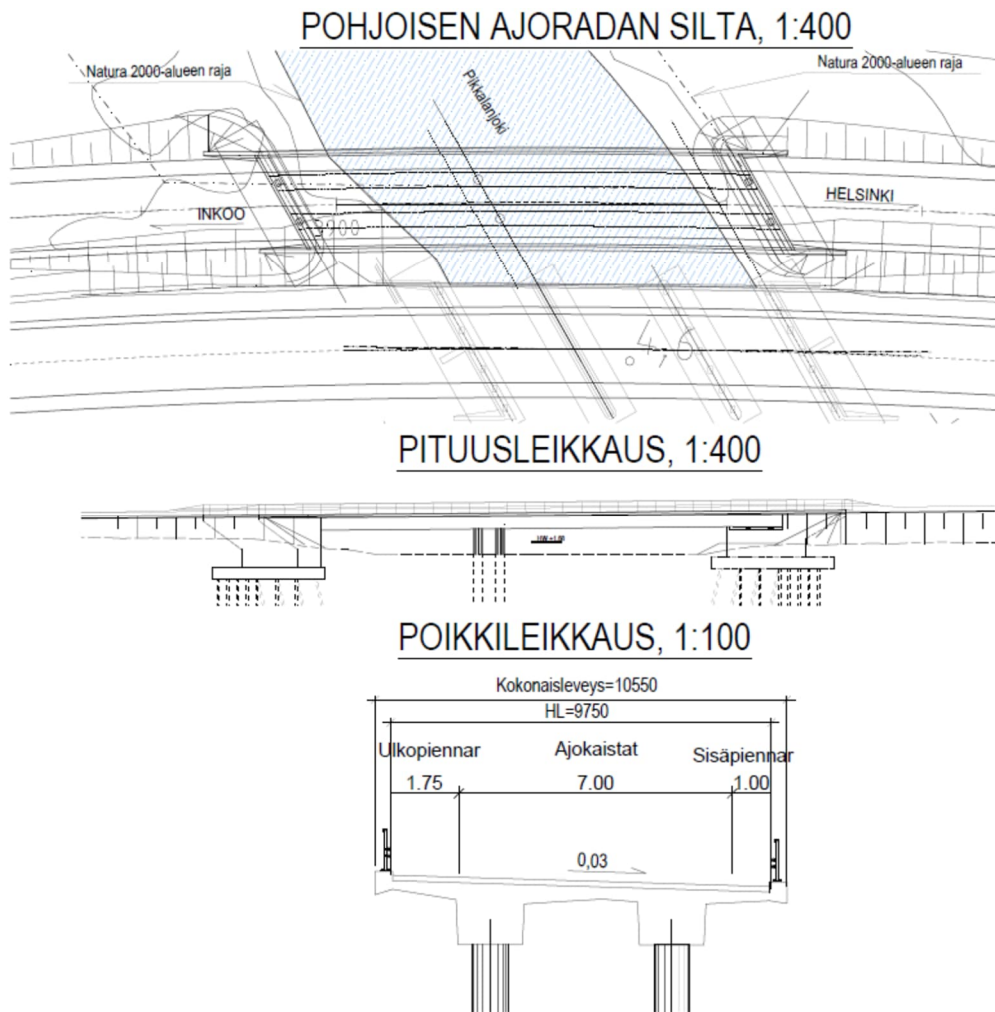
Kuva 6. Uuden Pikalanjoen sillan alustava pituus- ja poikkileikkaus.
