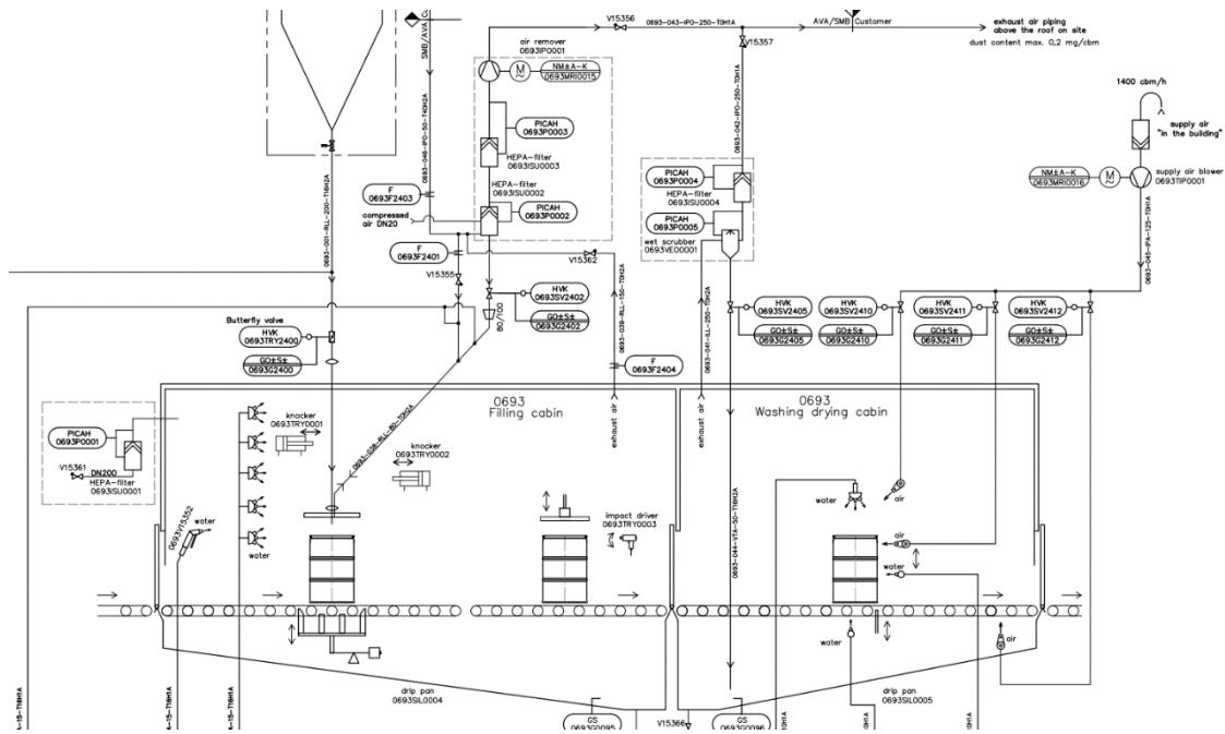
Kuva 2. Ilman kulku pakkauskontin ja HEPA-suodattimien kautta pois kuivaus- ja pakkaushallista.
