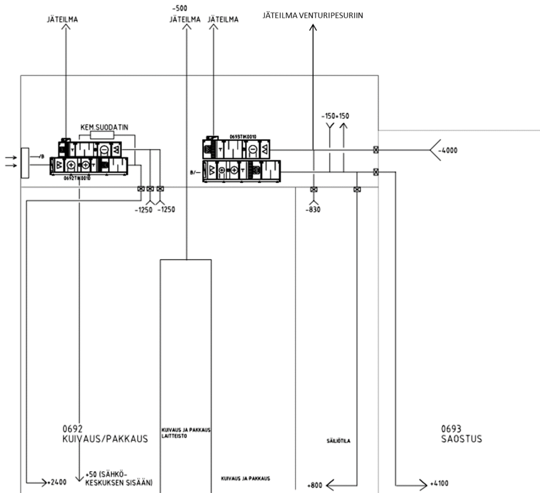
Kuva 1. Saostus-, kuivaus- ja pakkaushallien ilmastointijärjestelyn periaatekuva.
