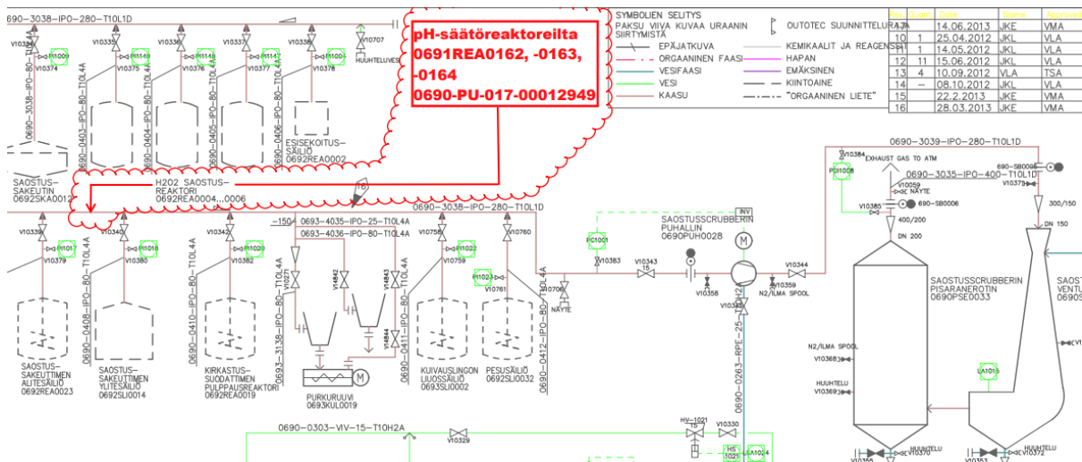
Kuva 3. pH:n säätöreaktoreista tuleva kostea, hiilidioksidipitoinen hönkäkaasu johdetaan saostushallin venturipesuriin. Kuvassa on esitetty muutos, joka on tehty saostushallin hönkien keruuputkistoon.
