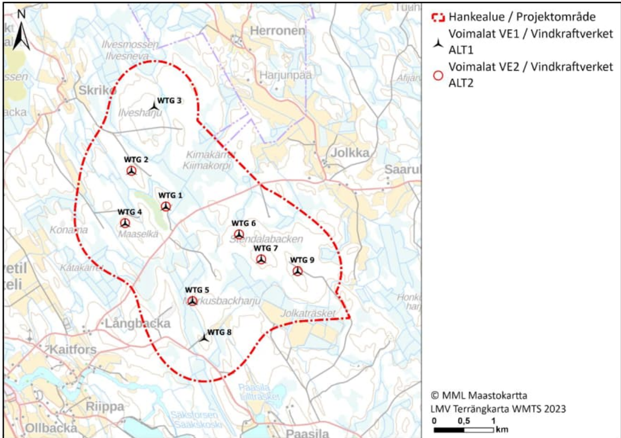
Kuva 4.1 Jolkan tuulivoimapaiston alustava voimalasijoittelu hankevaihtoehtoisissa VE1 ja VE2.
