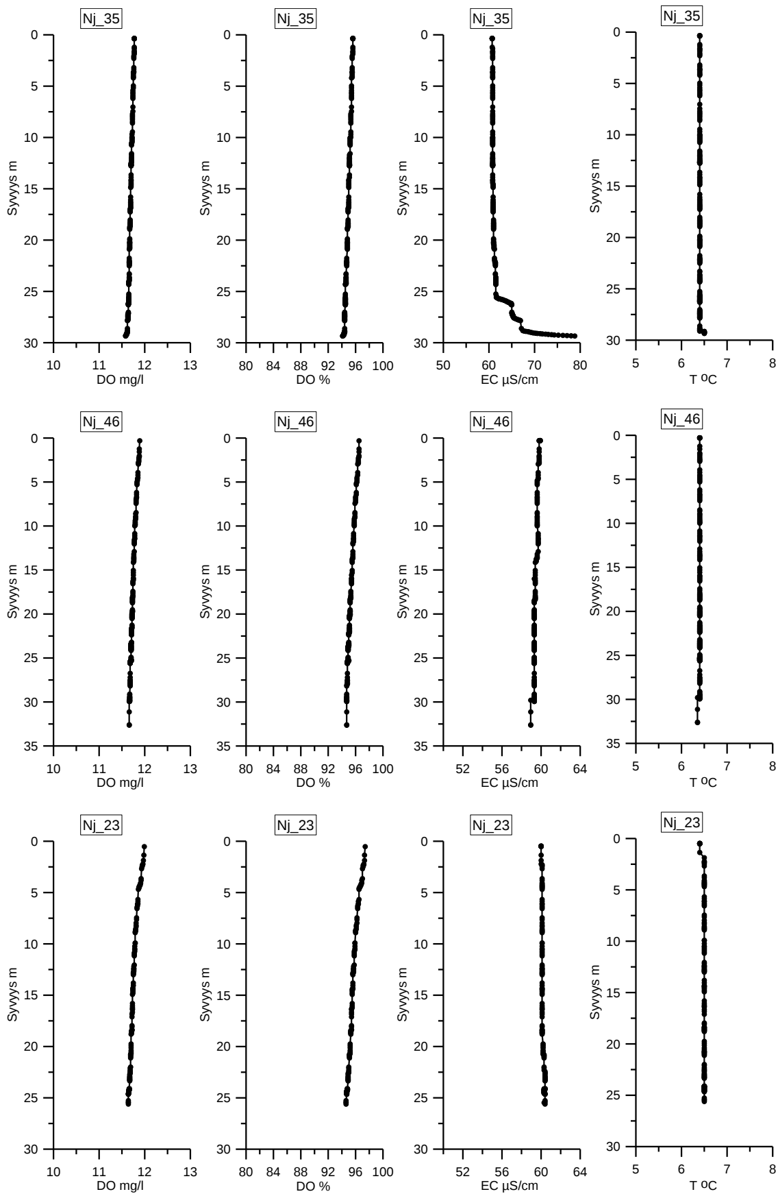
Kuva 1. Happipitoisuuden (DO mg/l), hapen kyllästysasteen (DO %), sähkönjohtavuuden (EC \mu\text{S/cm} ) ja lämpötilan (T ^{\circ}\text{C} ) vaihtelu syvyyden funktiona Nuasjäressä purkuputkesta 1-3 km etäisyydellä sijaitsevista syvänteistä Nj35, Nj46 ja Nj23. Tulokset ovat Geologian tutkimuskeskuksen mittauksista 20.–21.10.2016.
