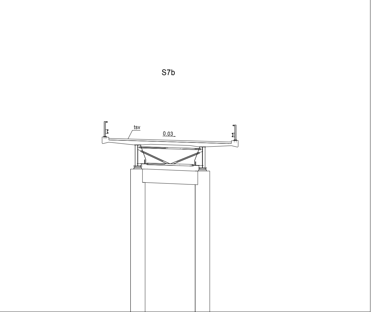
Leikkaus B-B 1:200
