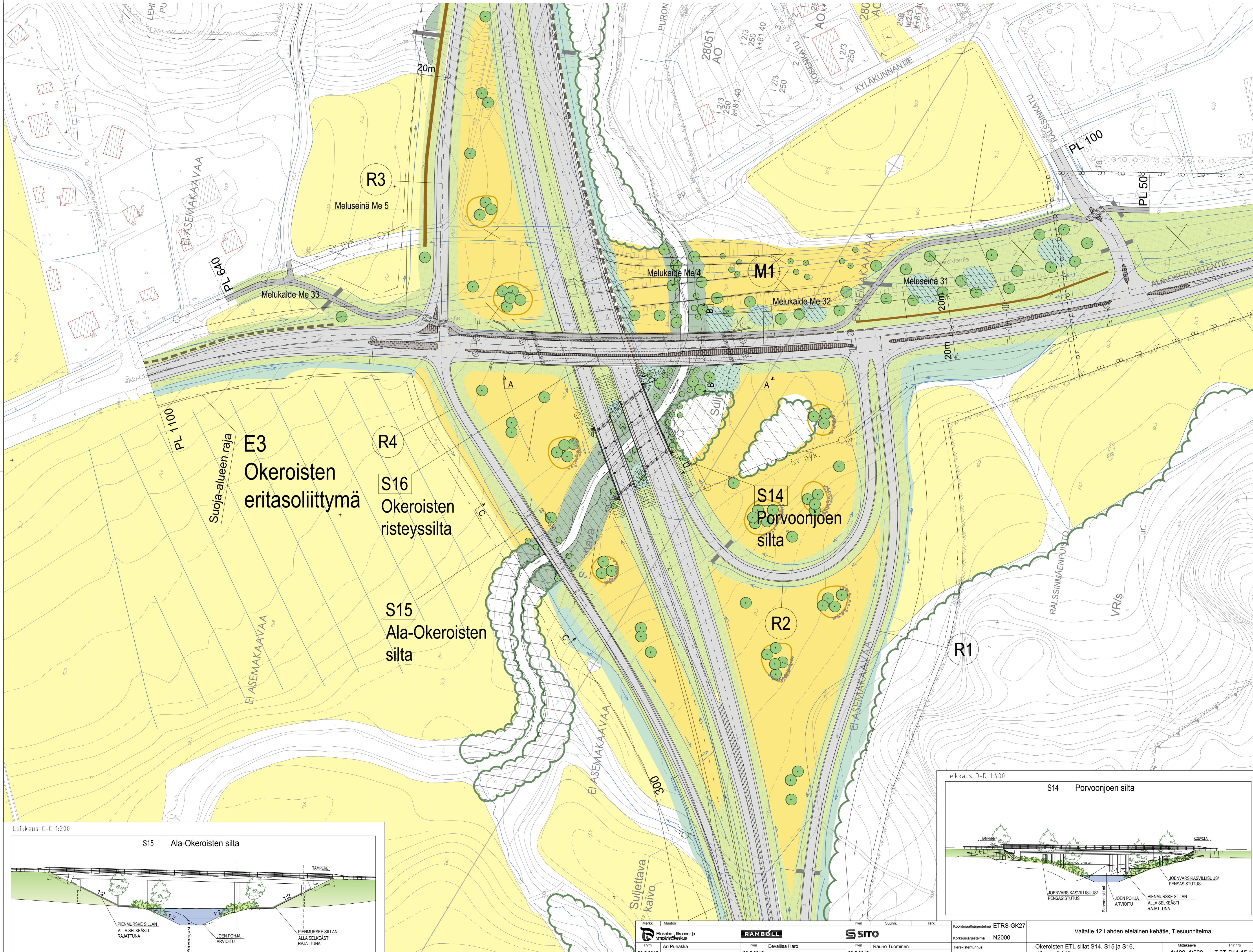
Tasokuva 1:1000
