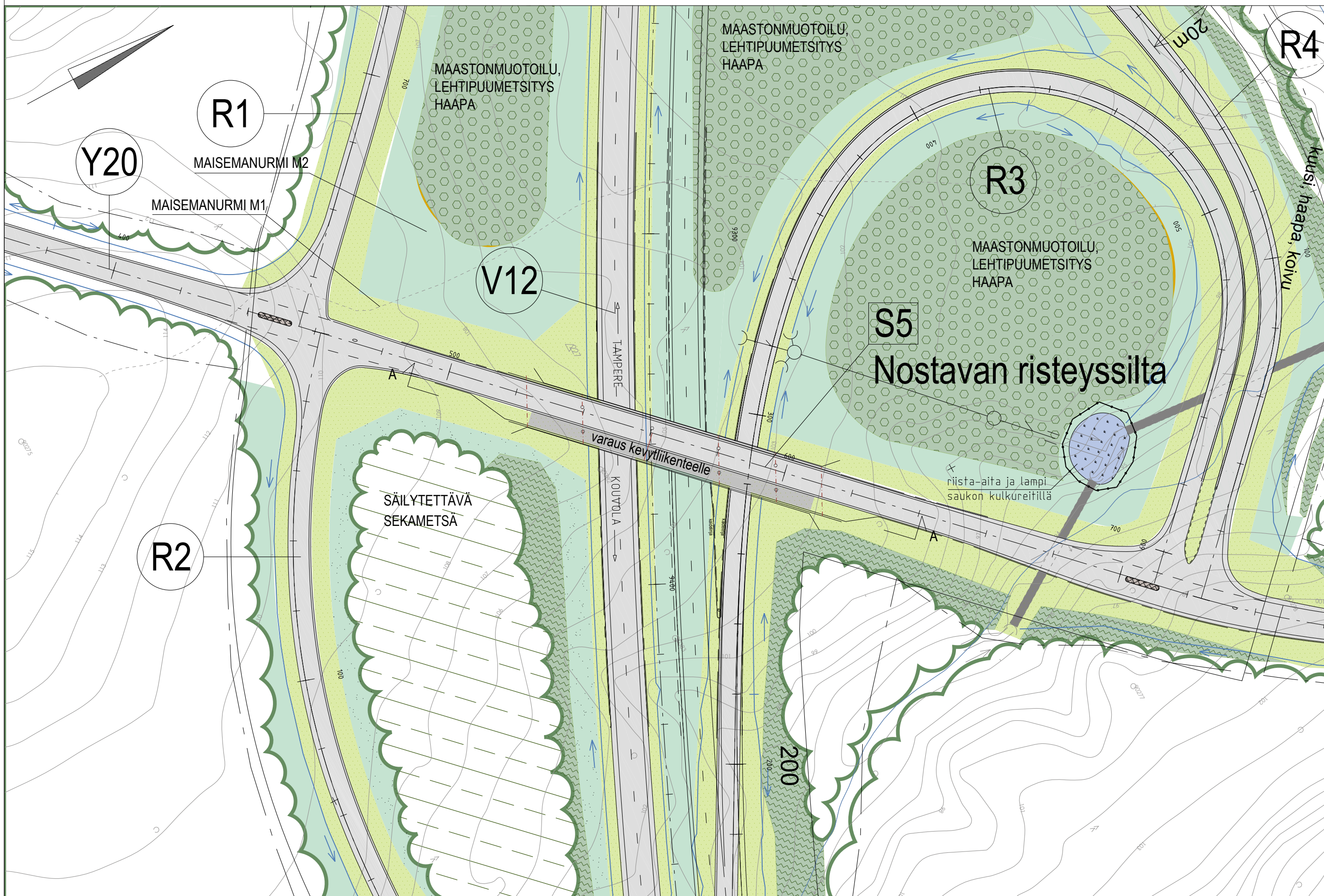
Tasokuva 1:400
