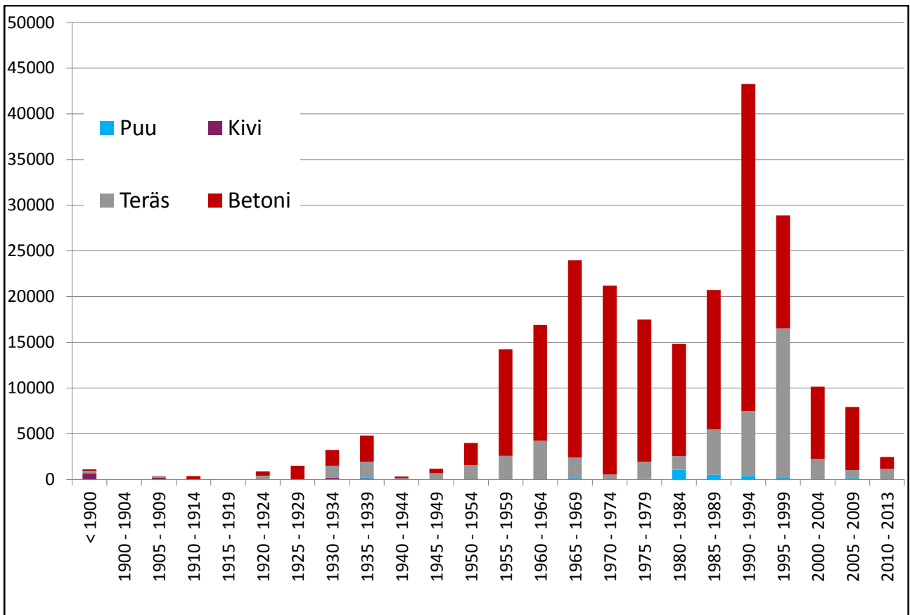
Etelä-Pohjanmaan ELY-keskuksen alueen valmistuneiden varsinaisten tiesiltojen kokonaispinta-alojen (m 2 ) ikäjakauma rakennusmateriaaleittain.
