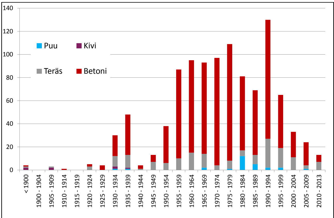
Etelä-Pohjanmaan ELY-keskuksen alueen valmistuneiden varsinaisten tiesiltojen lukumäärä (kpl) rakennusmateriaaleittain.
