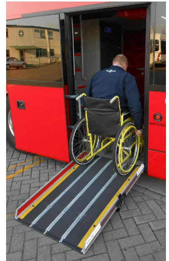
Kuvat 1 ja 2. Pyörätuoliramppi ja leveä ovi matalalattiaosastoon.
